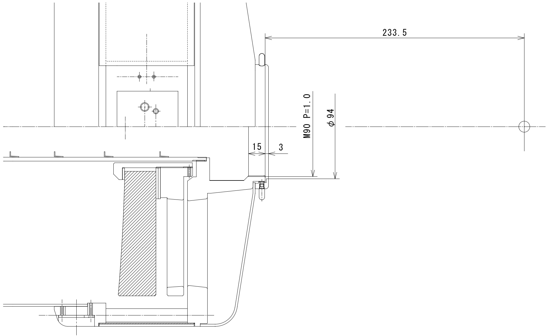
\mu - 300 接眼部取付け寸法図面
